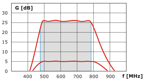
CHARAKTERYSTYKA CZĘSTOTLIWOŚCIOWA
